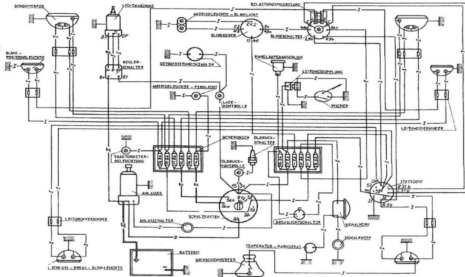
Schaltplan für FL 131 und FL 120
