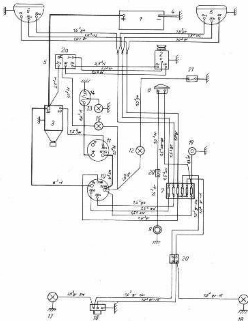
Bild 35 Schaltschema
